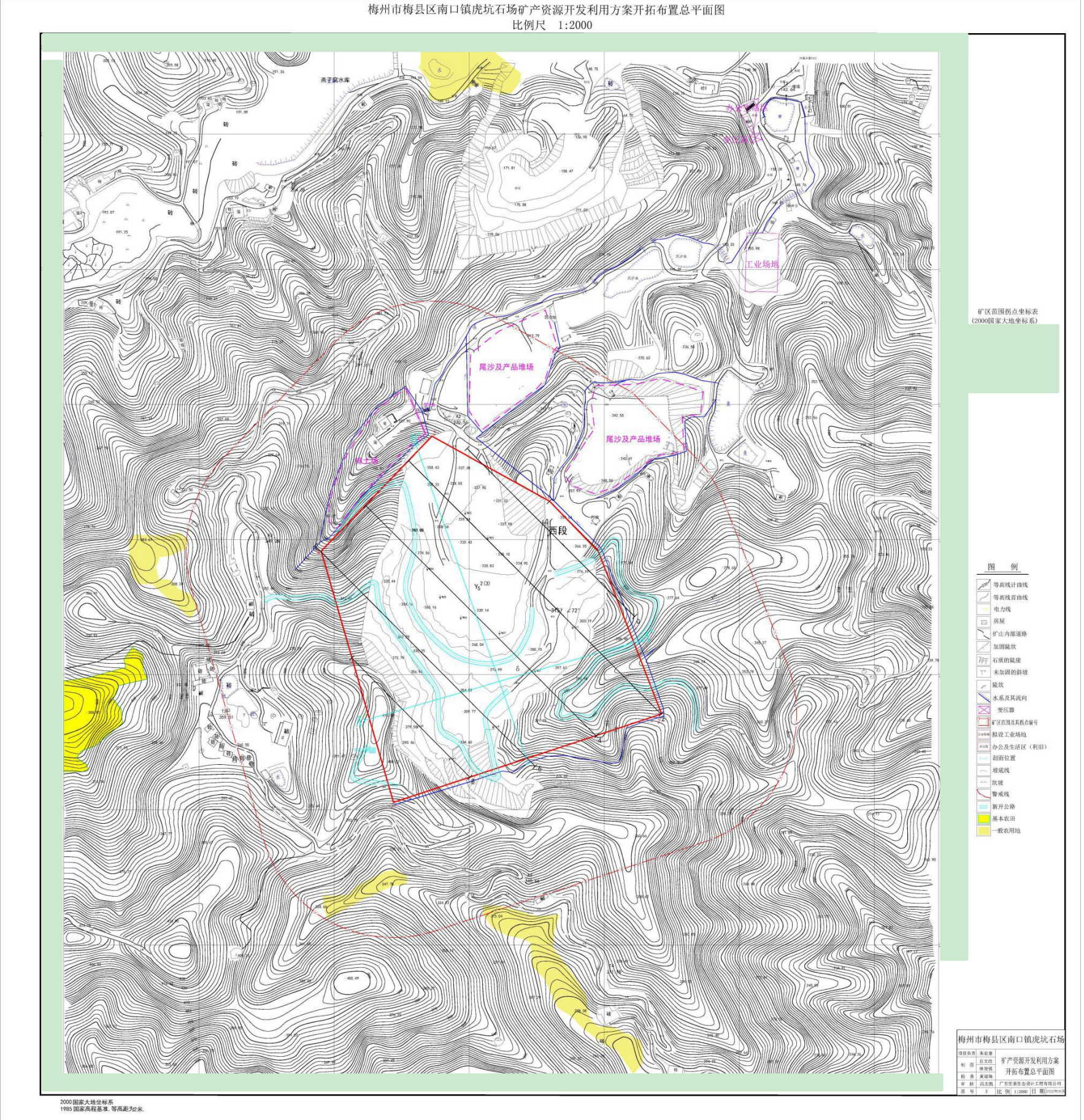
1-3 开拓布置总平面图
