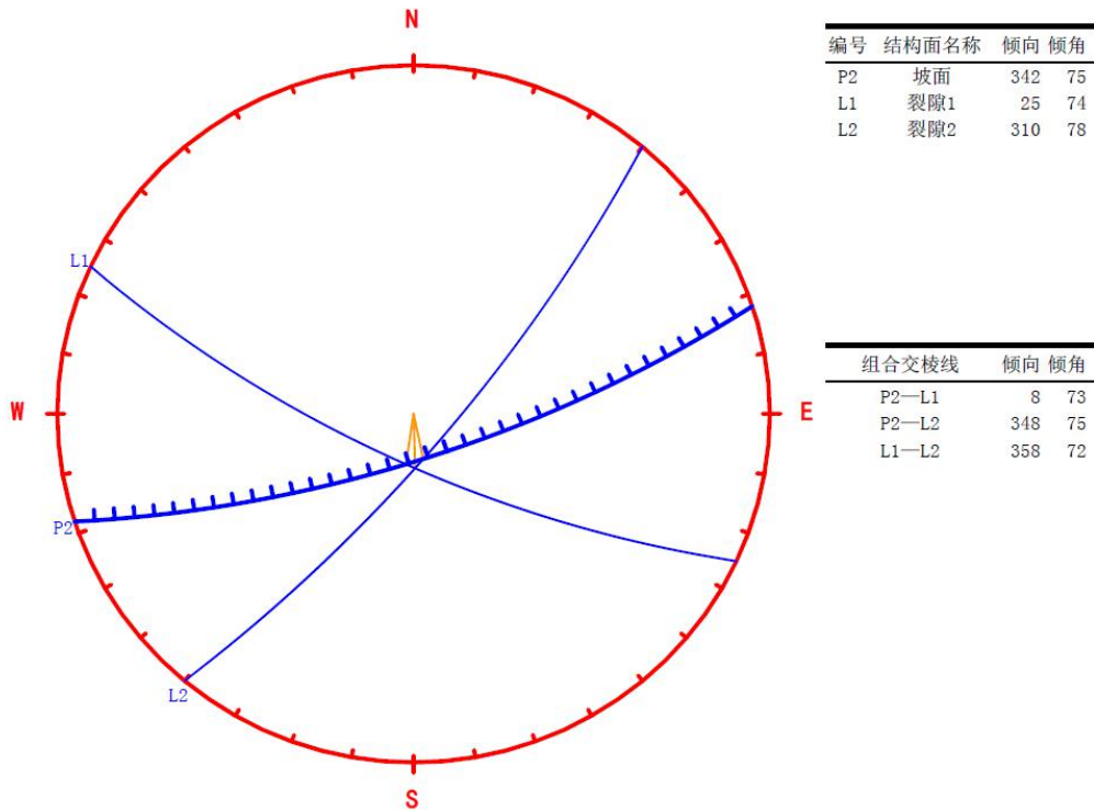
图 3-2 东南侧边坡赤平投影
